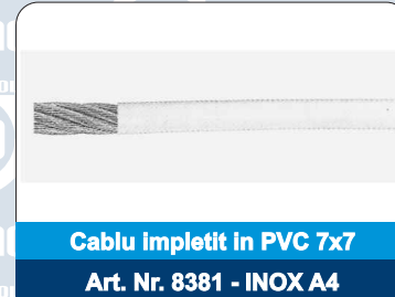
Cablu impletit in PVC 7x7 Art. Nr. 8381 - INOX A4
